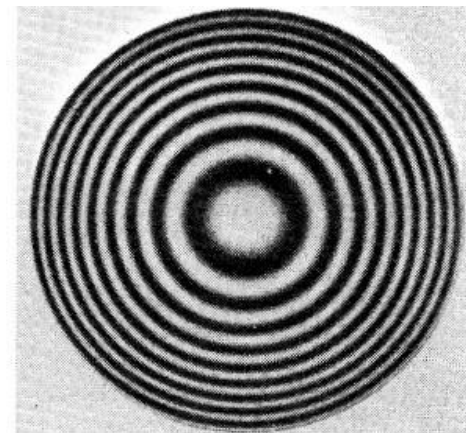
Figura di interferenza da fenditura circolare
